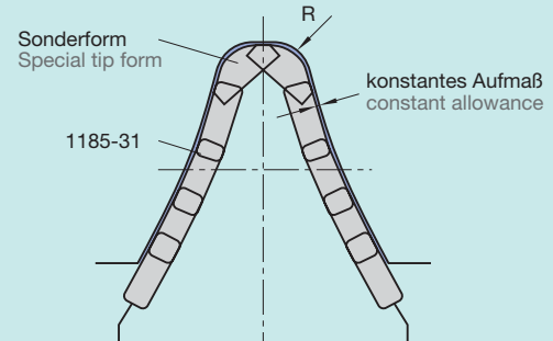
Abb. 3 Sonderprofil
