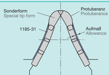
Abb. 4 Sonderprofil
