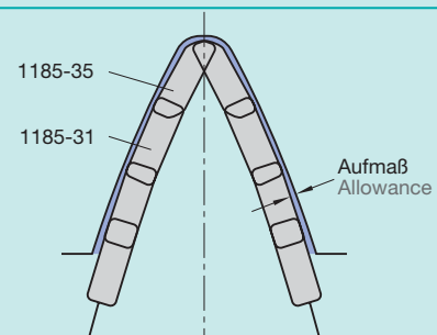
Abb. 5 Sonderprofil
