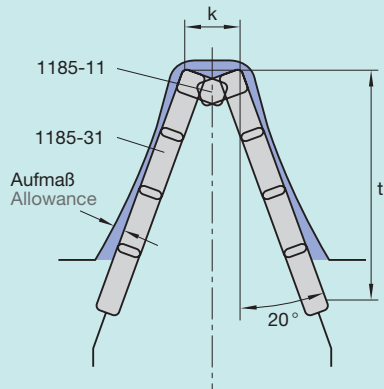
Abb. 1 Standard-Ausführung
